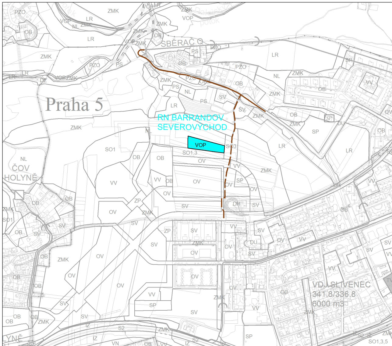
Návrh změny, výkres č.9 - Vodní hospodářství a odpady
