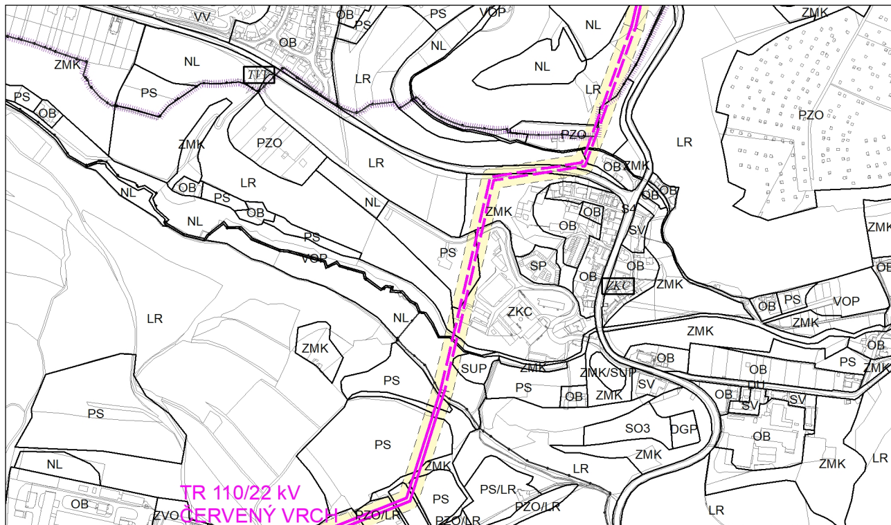
Výkres č. 10 – Energetika, platný stav k 1. 1. 2020
