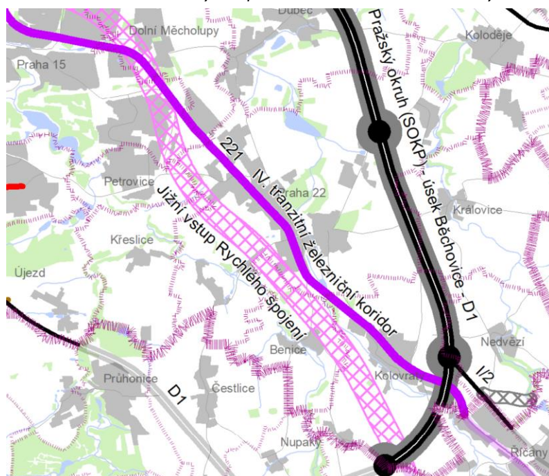
Obrázek 5: Výkres plocha a koridorů nadmístního významu – dopravní infrastruktura
