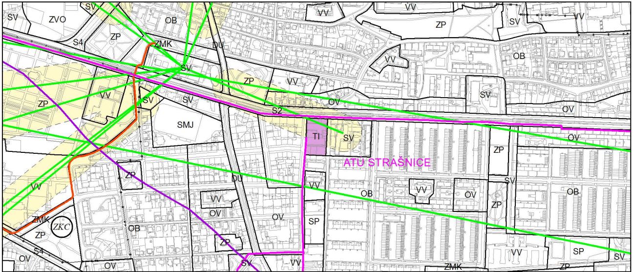
Výkres č. 11 – Přenos informací a kolektory, platný stav k 1. 1. 2017
