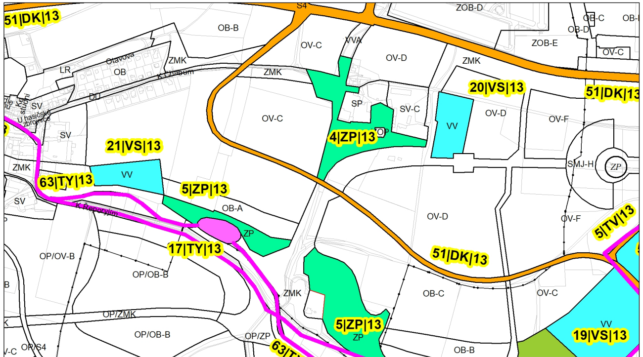
Výkres č. 25 – Veřejně prospěšné stavby, platný stav k 17. 6. 2021
