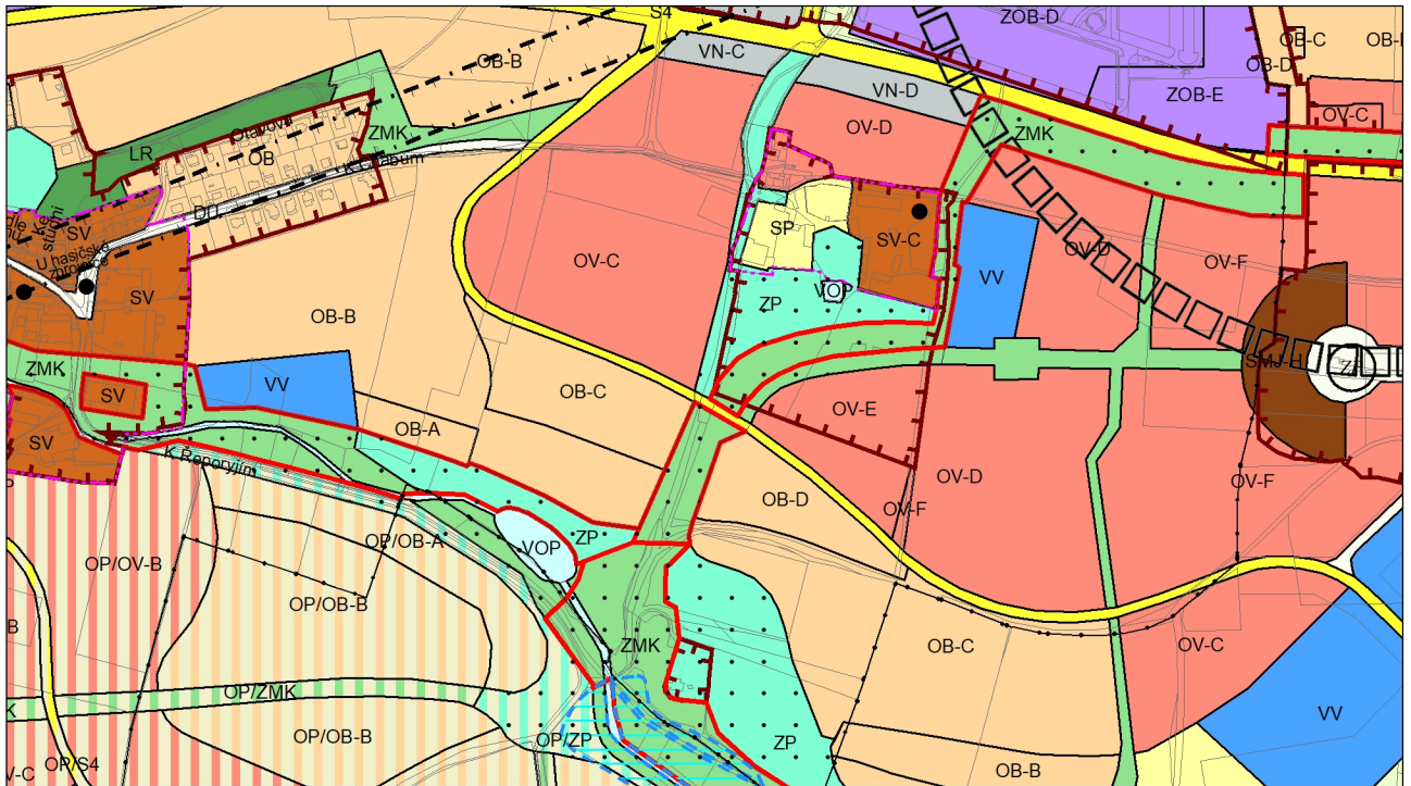
Promítnutí změny do výkresu č. 4 - Plán využití ploch, platný stav k 17. 6. 2021
