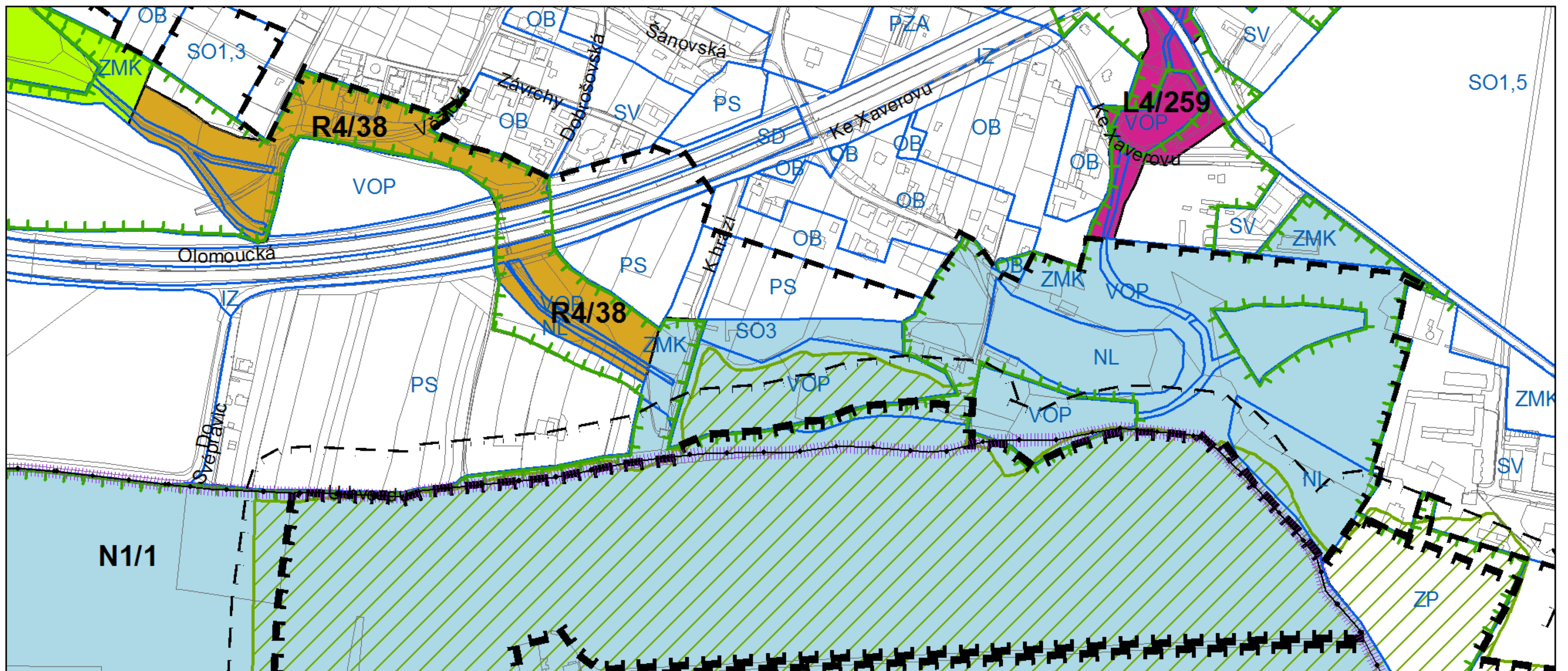
Výkres č. 19 – Územní systém ekologické stability, platný stav k 1. 1. 2018
