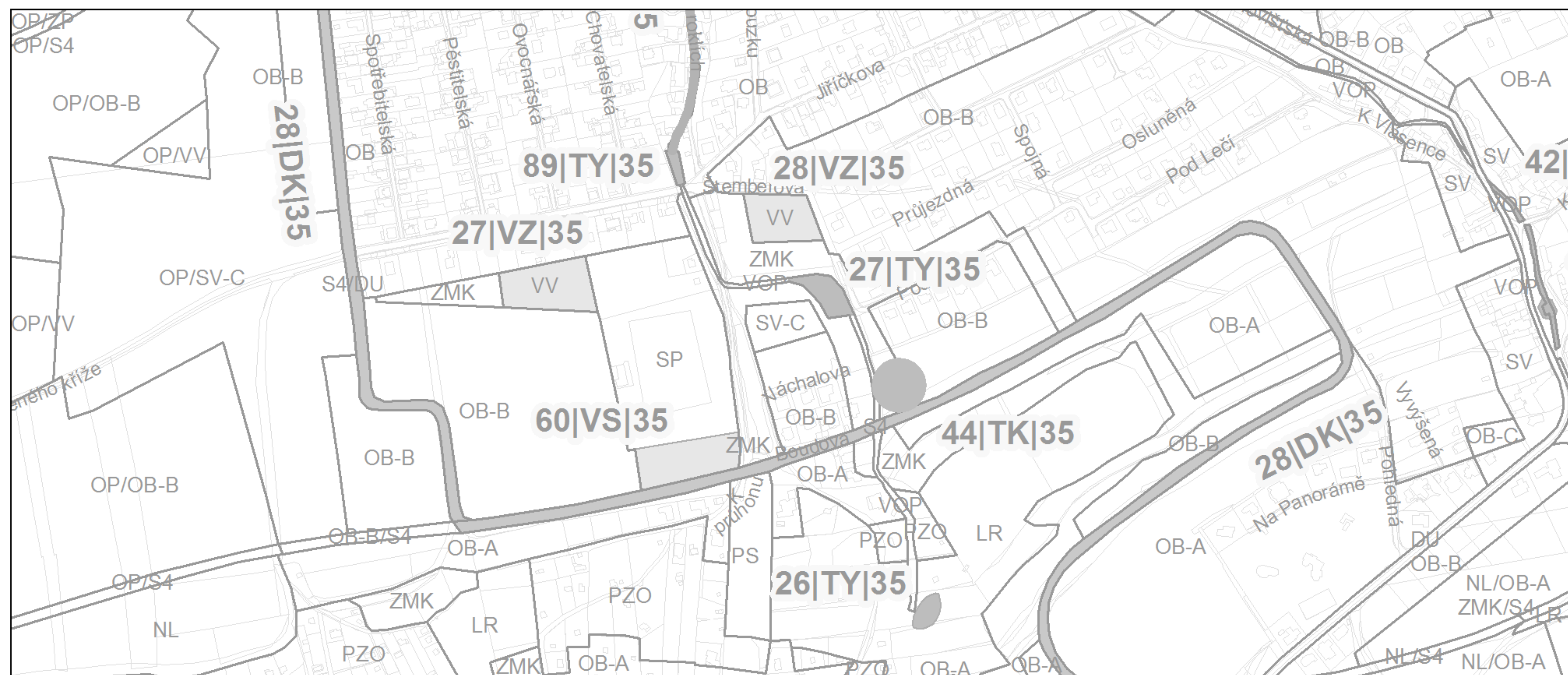
Návrh změny, výkres č. 5 – Veřejně prospěšné stavby
