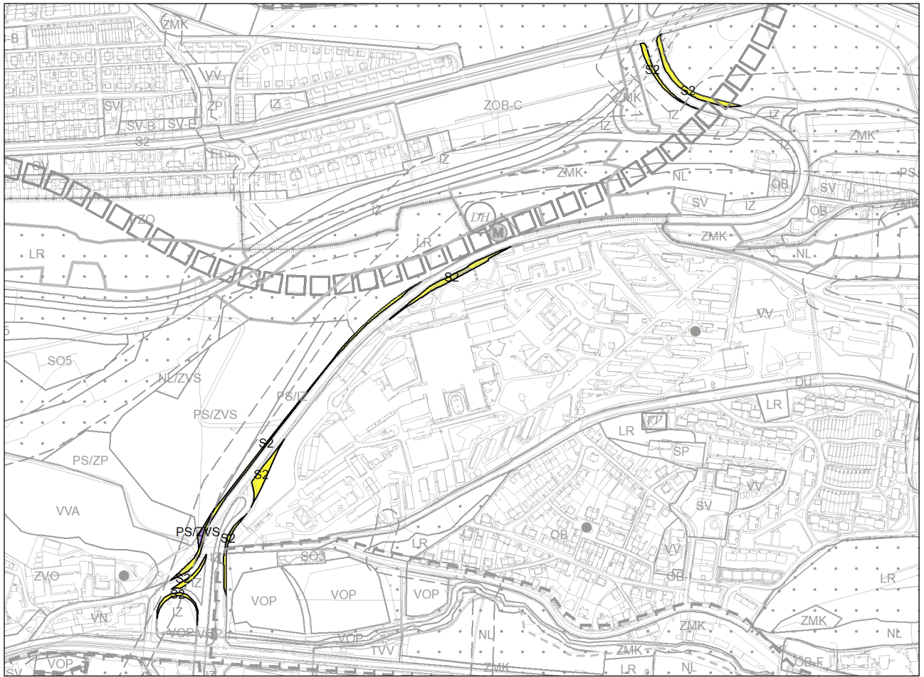
Návrh změny, výkres č. 4 – Plán využití ploch
