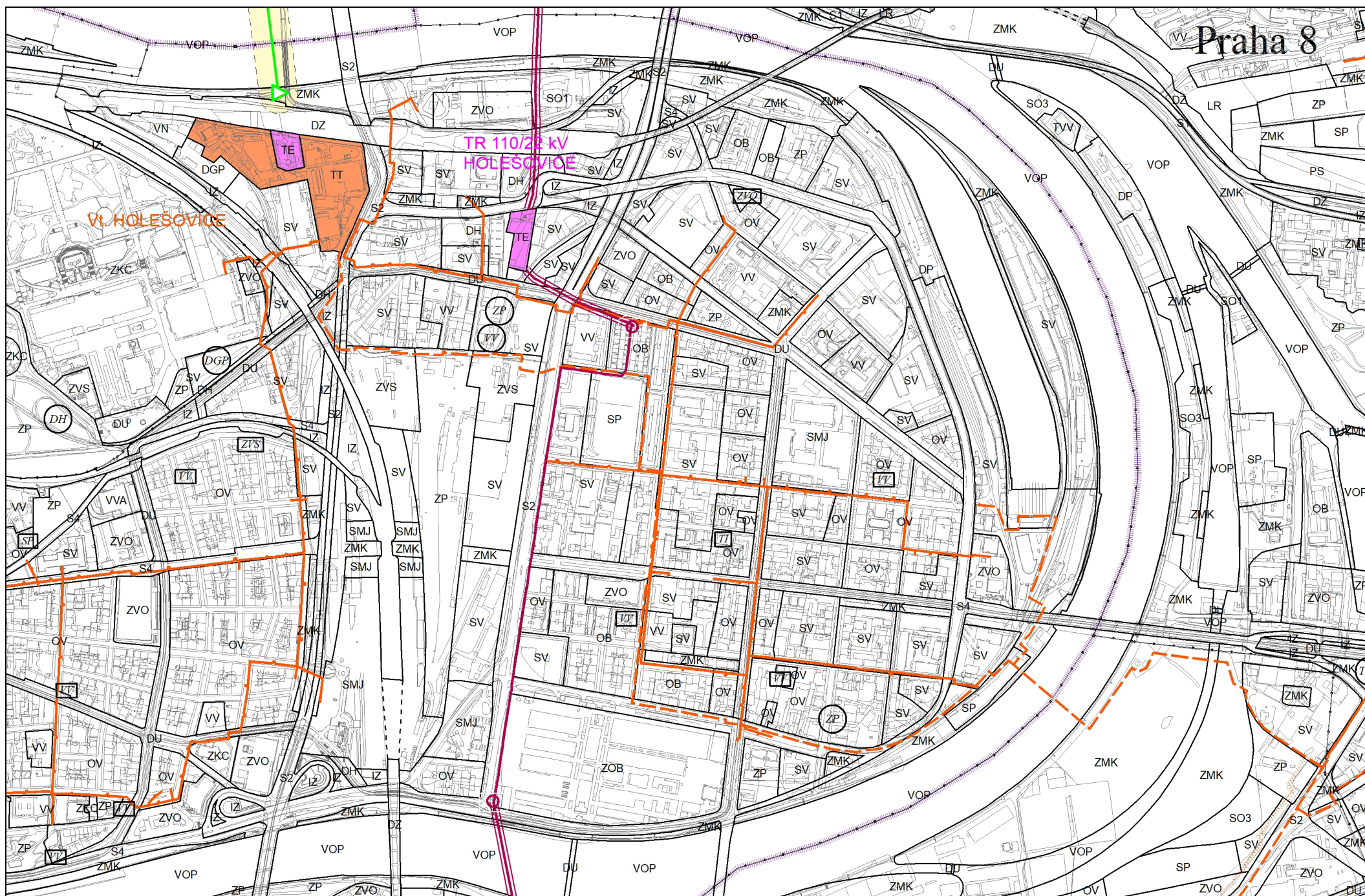
Výkres č. 10 – Energetika, platný stav k 1. 1. 2020
