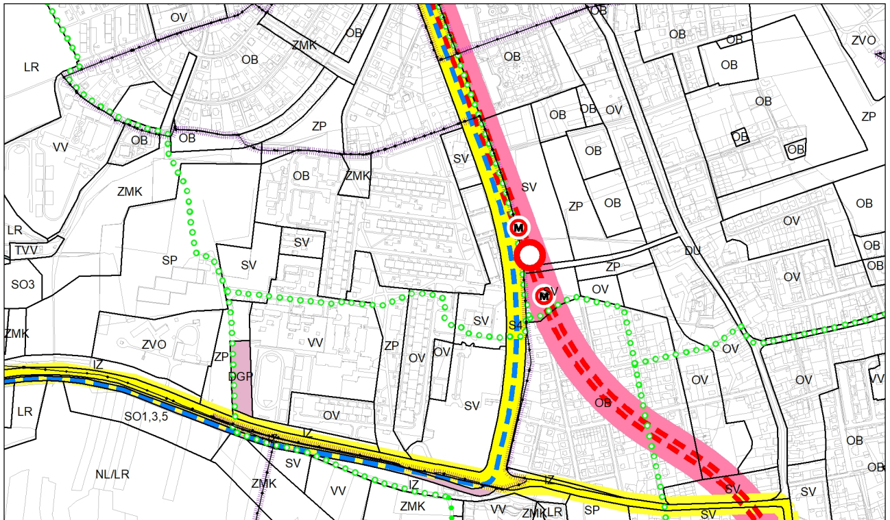
Výkres č. 5 – Doprava, platný stav k 17. 6. 2021
