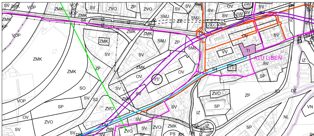
Výkres č. 11 – Přenos informací a kolektory, platný stav k 17. 6. 2021
