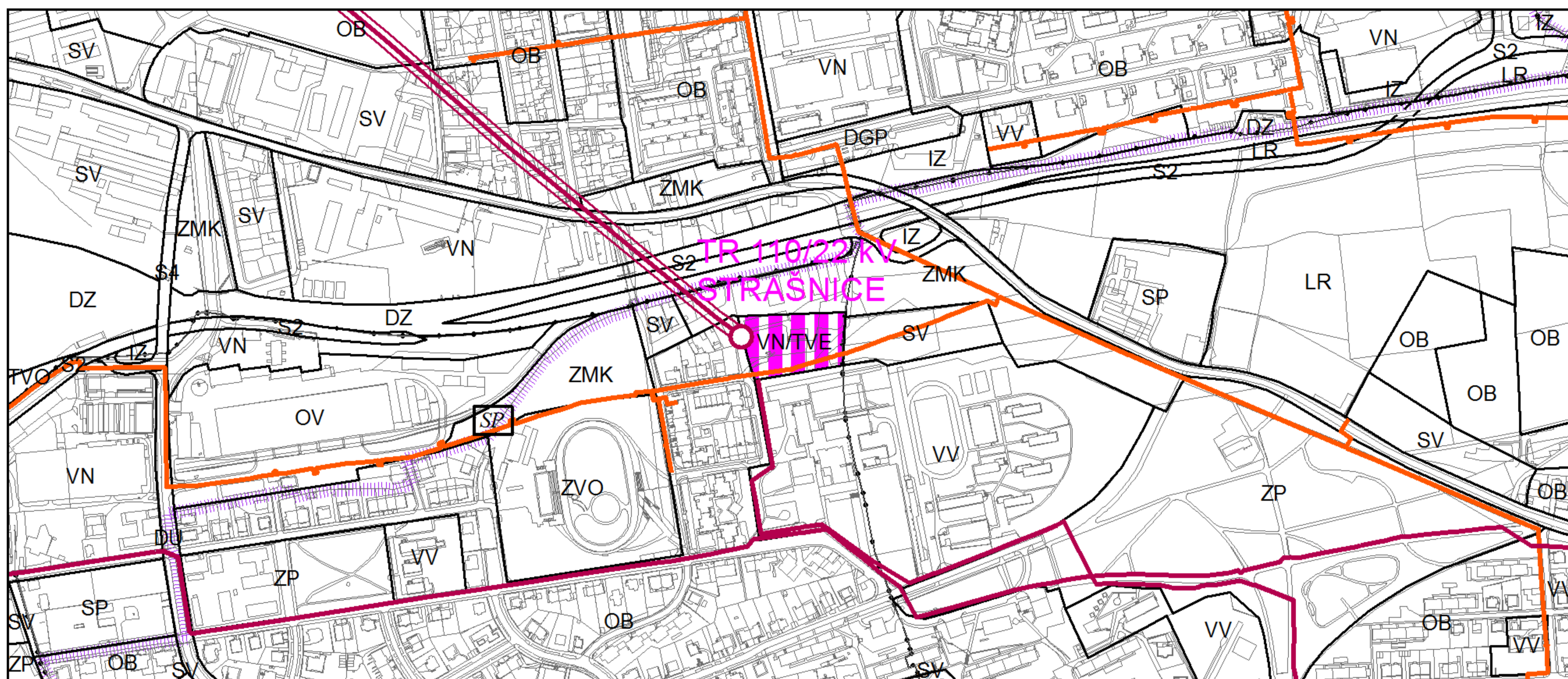
Výkres č. 10 – Energetika, platný stav k 1. 1. 2017
