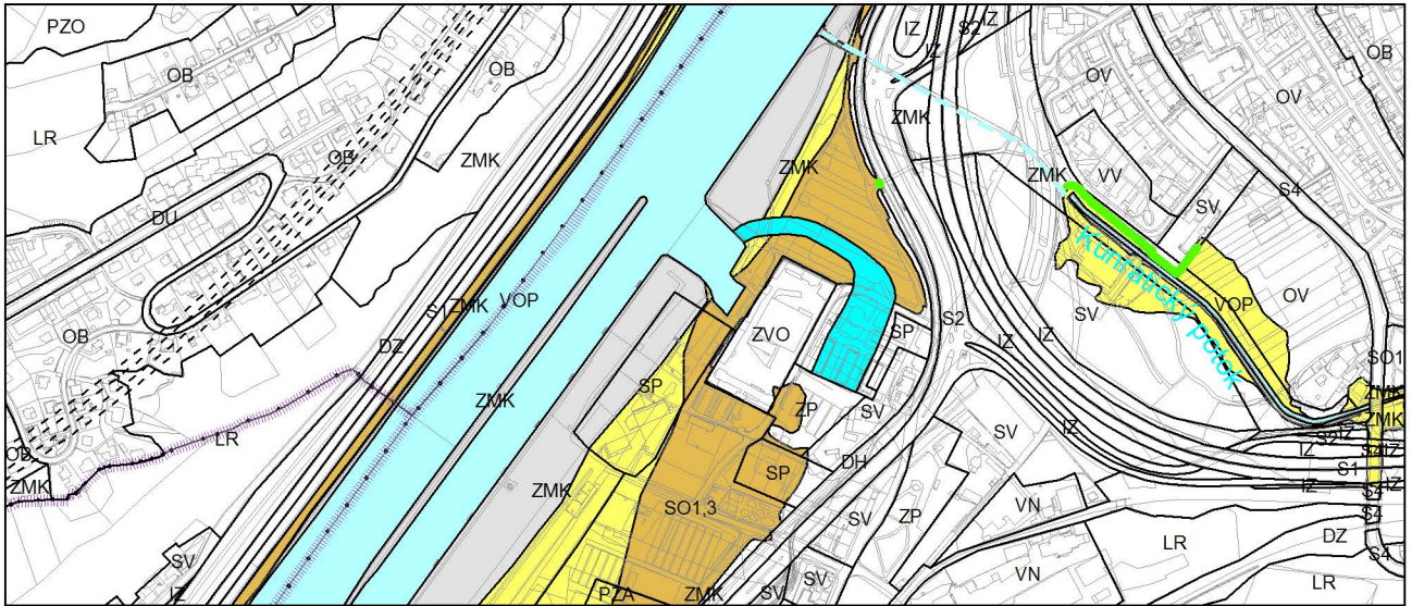
Výkres č. 33 – Kategorizace záplavových území, platný stav k 12. 1. 2016
