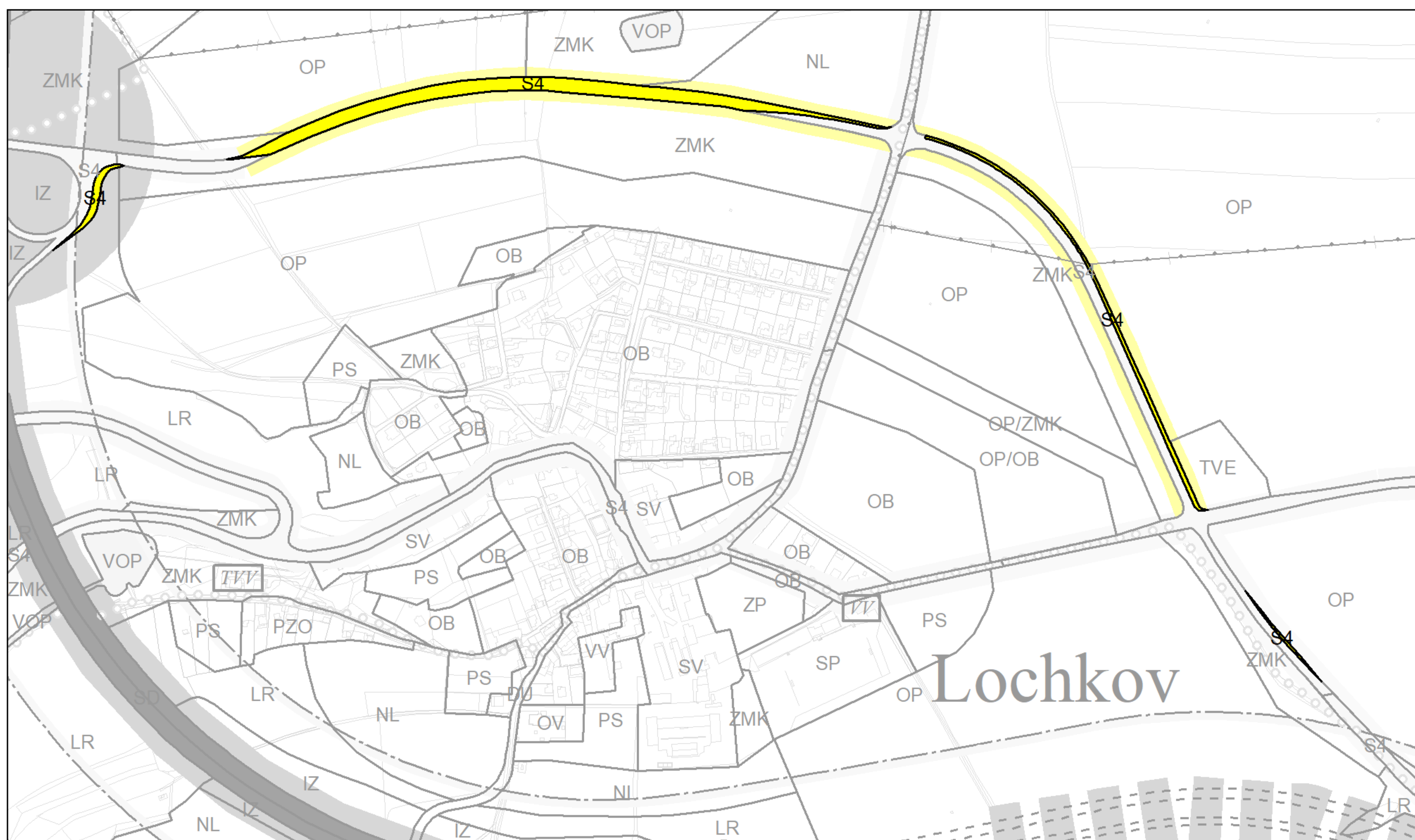
Návrh změny, výkres č. 5 – Doprava
