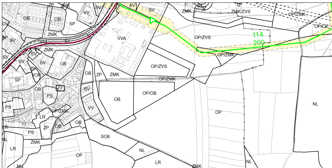
Výkres č. 10 – Energetika, platný stav k 8. 9. 2022
