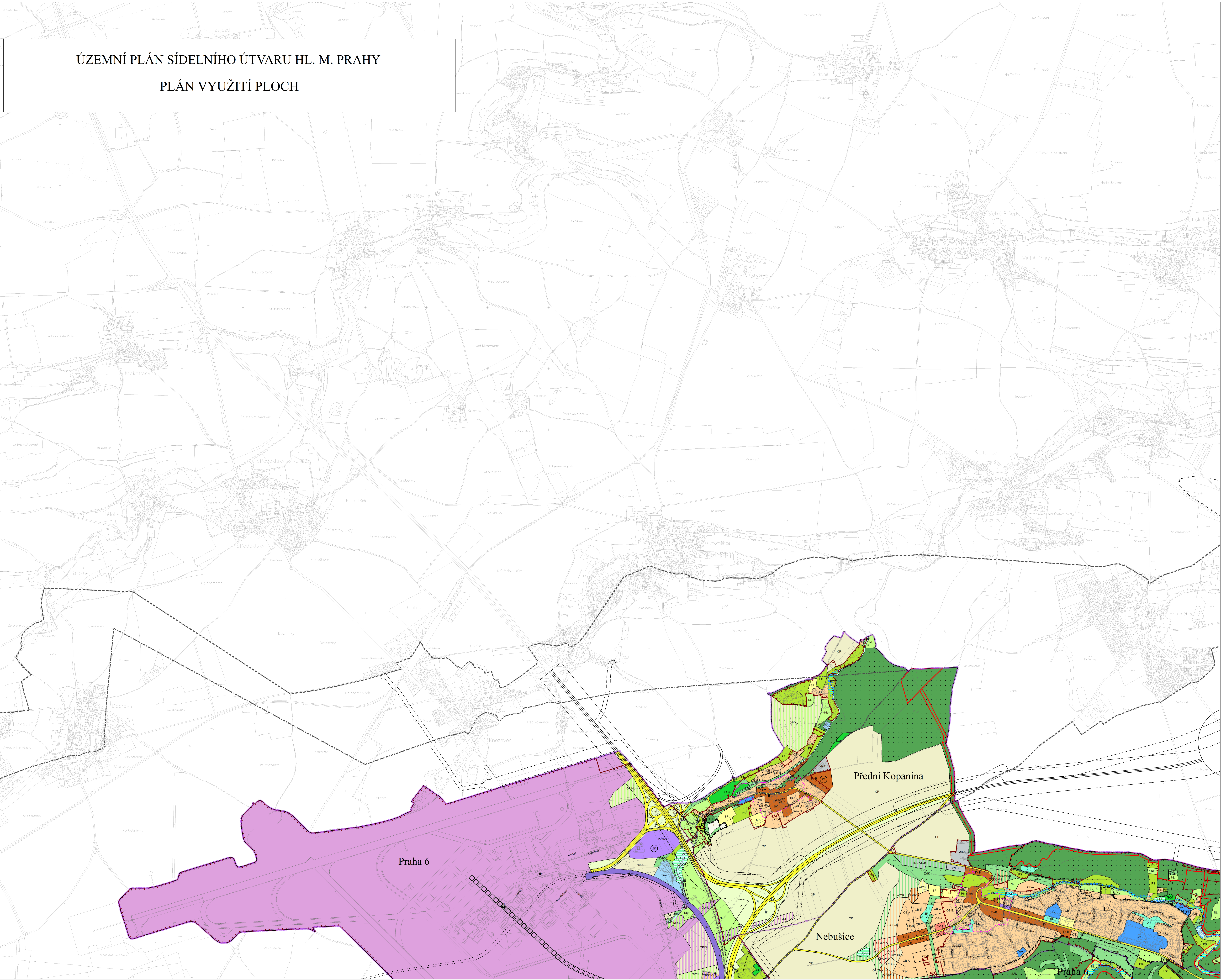
VÝKRES č. 4 - PLÁN VYUŽITÍ PLOCH MĚRÍTKO 1 : 10 000 (c) Institut plánování a rozvoje hl. m. Prahy, 2025
