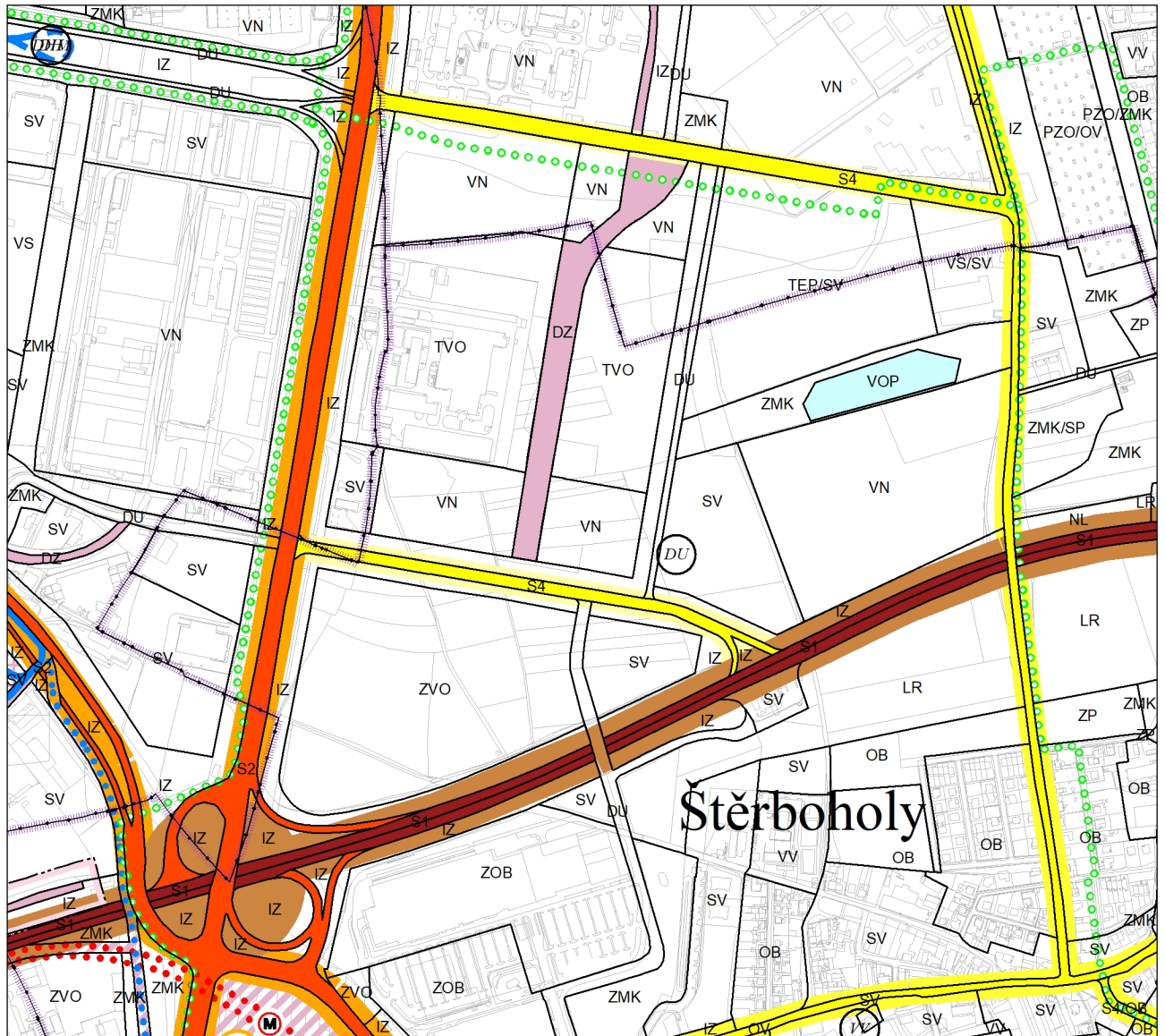
Promítnutí změny do výkresu č. 5 – Doprava, platný stav k 1. 1. 2022
