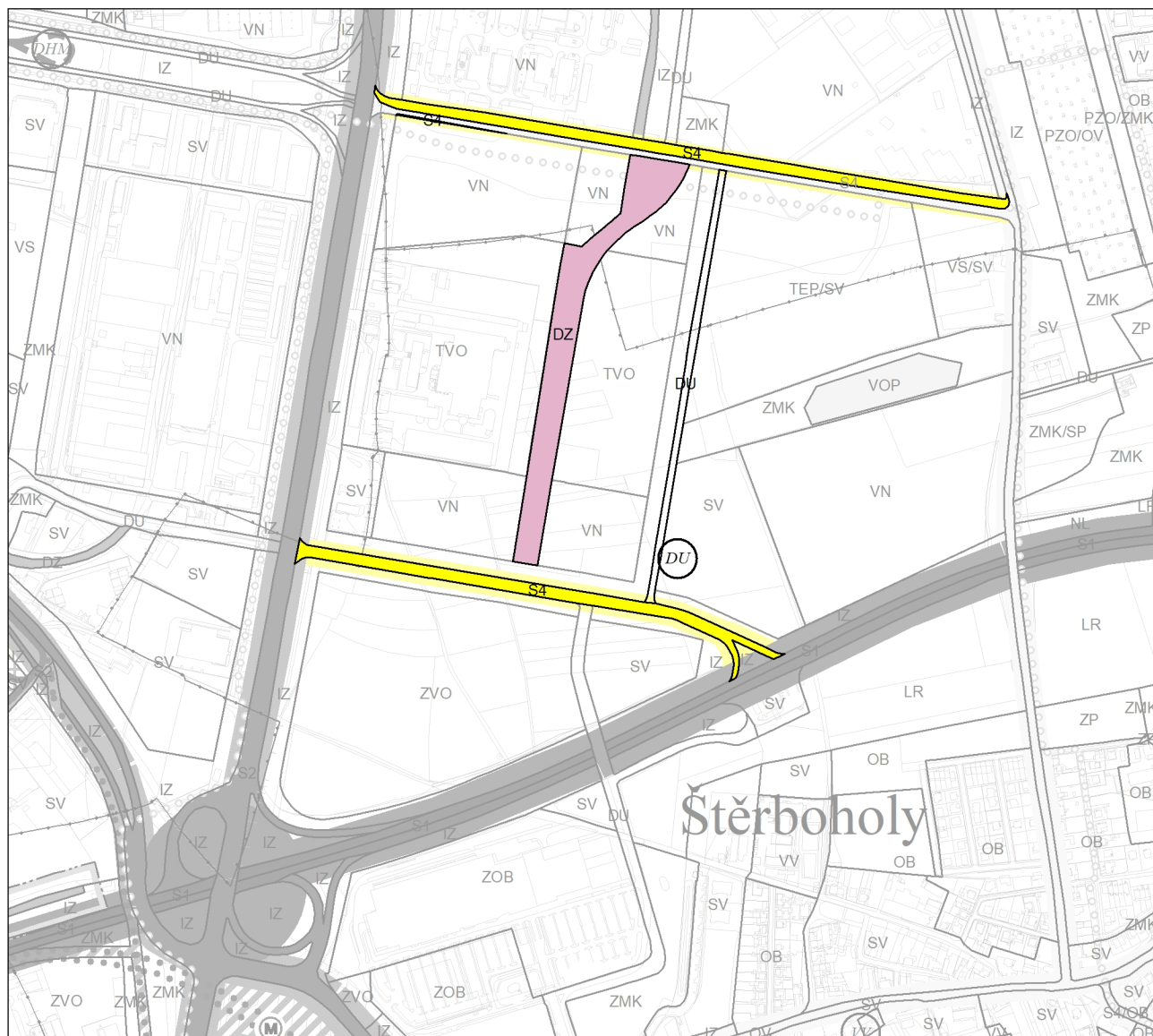
Návrh změny, výkres č. 5 – Doprava
