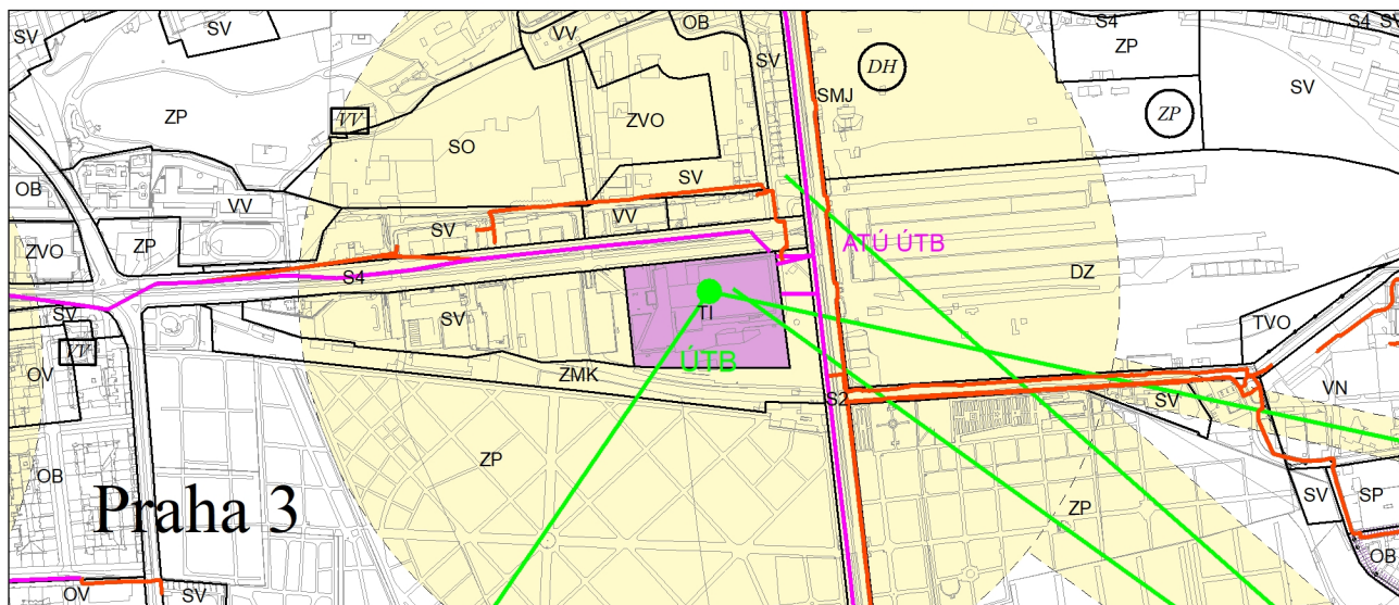
Výkres č. 11 – Přenos informací a kolektory, platný stav k 1. 1. 2018
