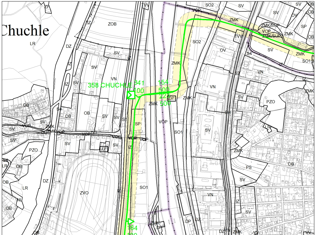
Výkres č. 10 – Energetika, platný stav k 1. 1. 2020
