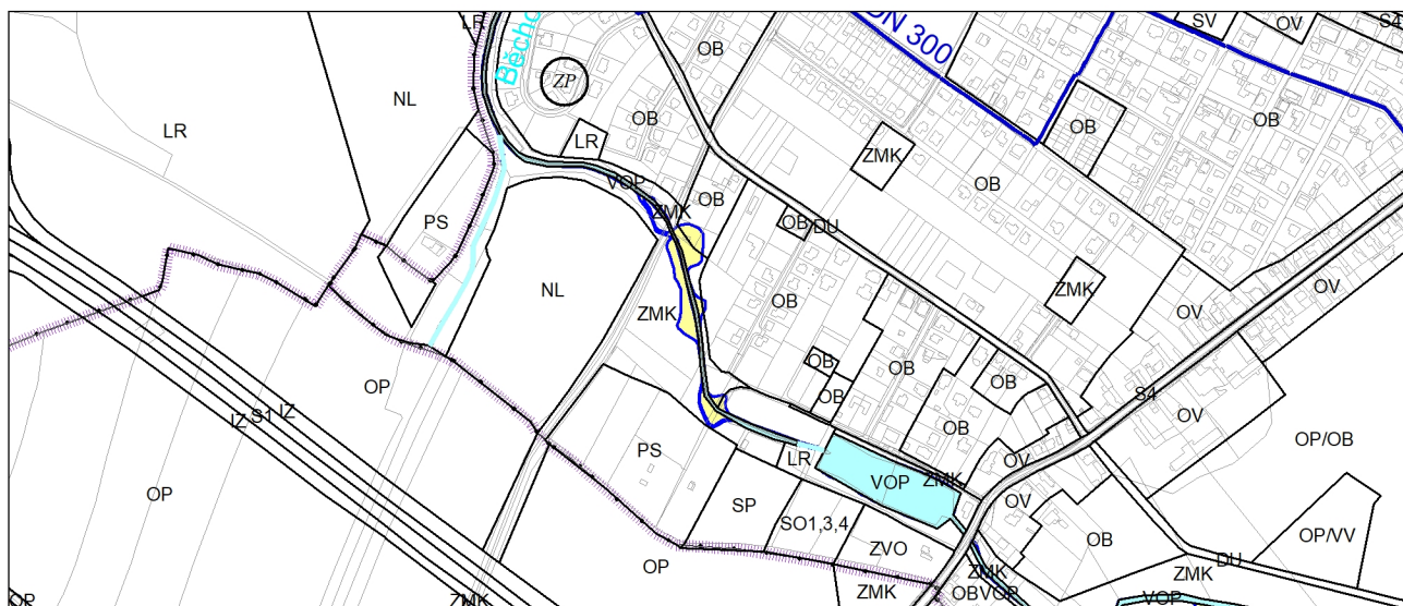
Promítnutí změny do výkresu č. 9 – Vodní hospodářství a odpady, platný stav k 1. 1. 2020
