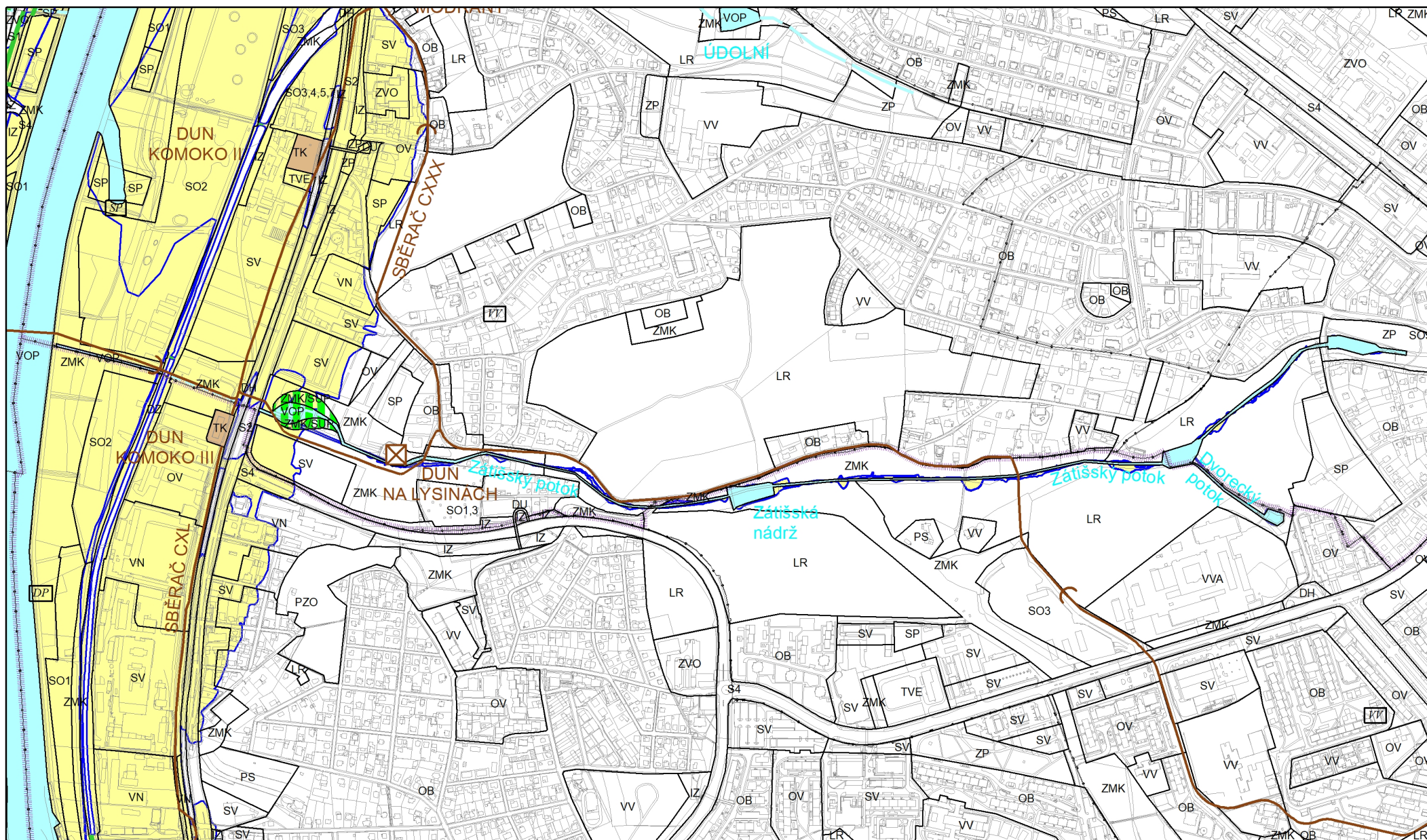
Promítnutí změny do výkresu č. 9 - Vodní hospodářství a odpady, platný stav k 1. 1. 2020
