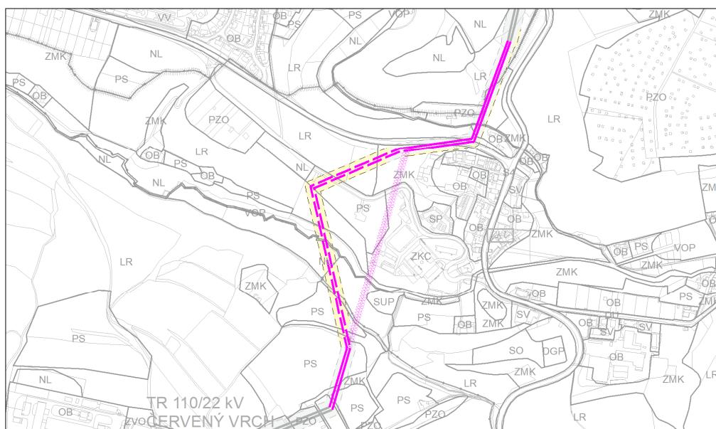
Ilustrační výřez výkresu č. 10 Energetika
